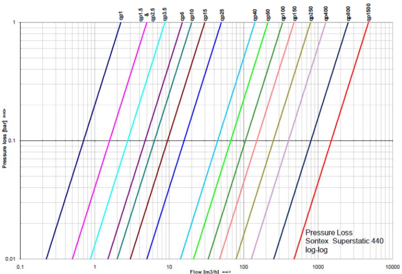
Druckverlustkurve
